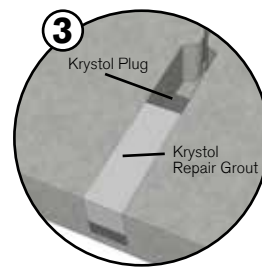
使用凯顿的裂缝修补系统修复渗漏裂缝
