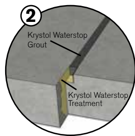
使用Krystol®止水带系统建筑密不透水的施工缝
